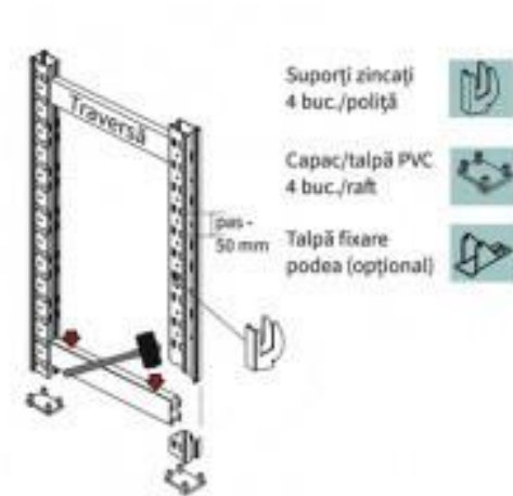
Traverse rigidizare
